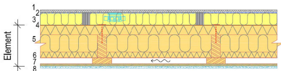
Схема 3. Типы внешних стен
